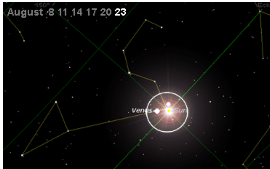
Regulus-Soleil (Sun)-Vénus-Jupiter
