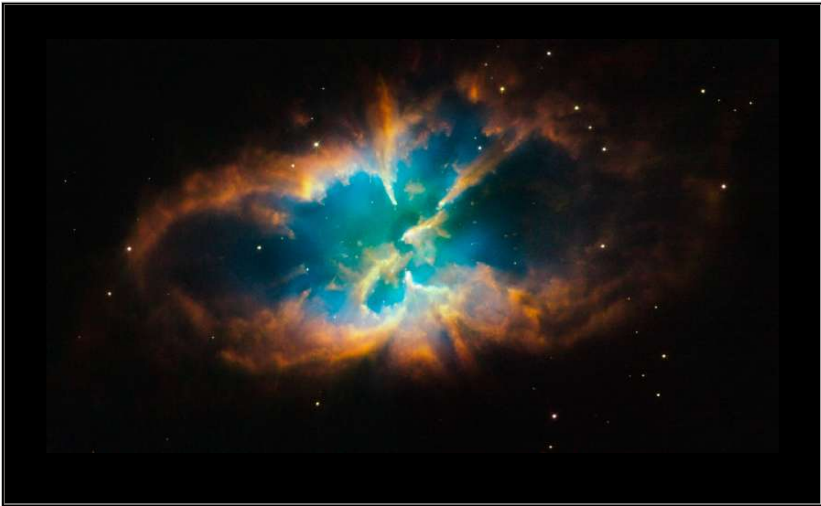
NGC 2818 vu par Hubble
