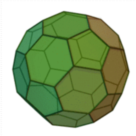
icosaèdre tronqué
