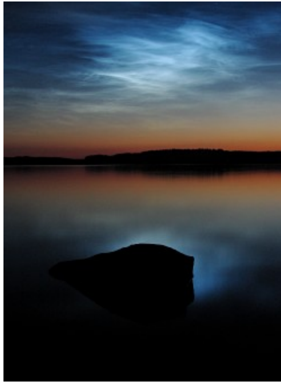
Image de Mika Yrjölä - Août 2003. nuage noctilucent au-dessus du lac Saimaa
