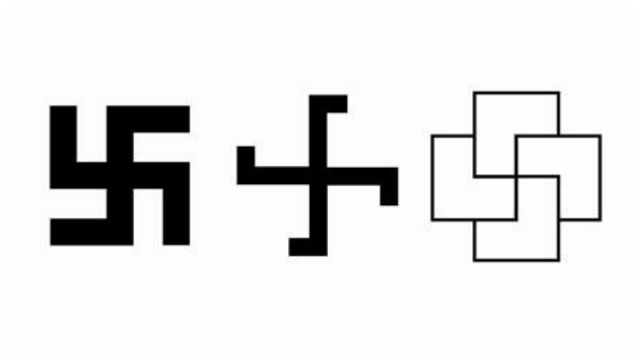
Swastikas
