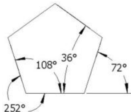
Valeurs angulaires d'un Pentagone
